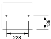
Gehäusezeichnungen mit Schraubpunkten zum Aufhängen der Quader-10 enclosure drawings with screwpoints for hanging the Quader-10
